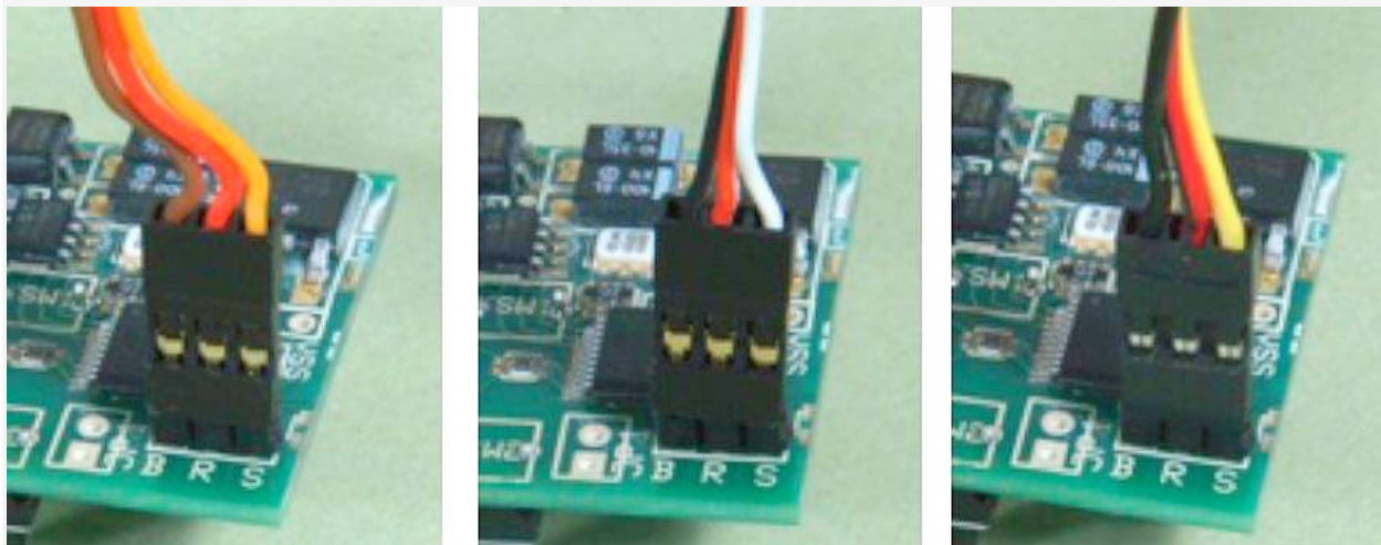
Servokabel - Farbenzuordnung
